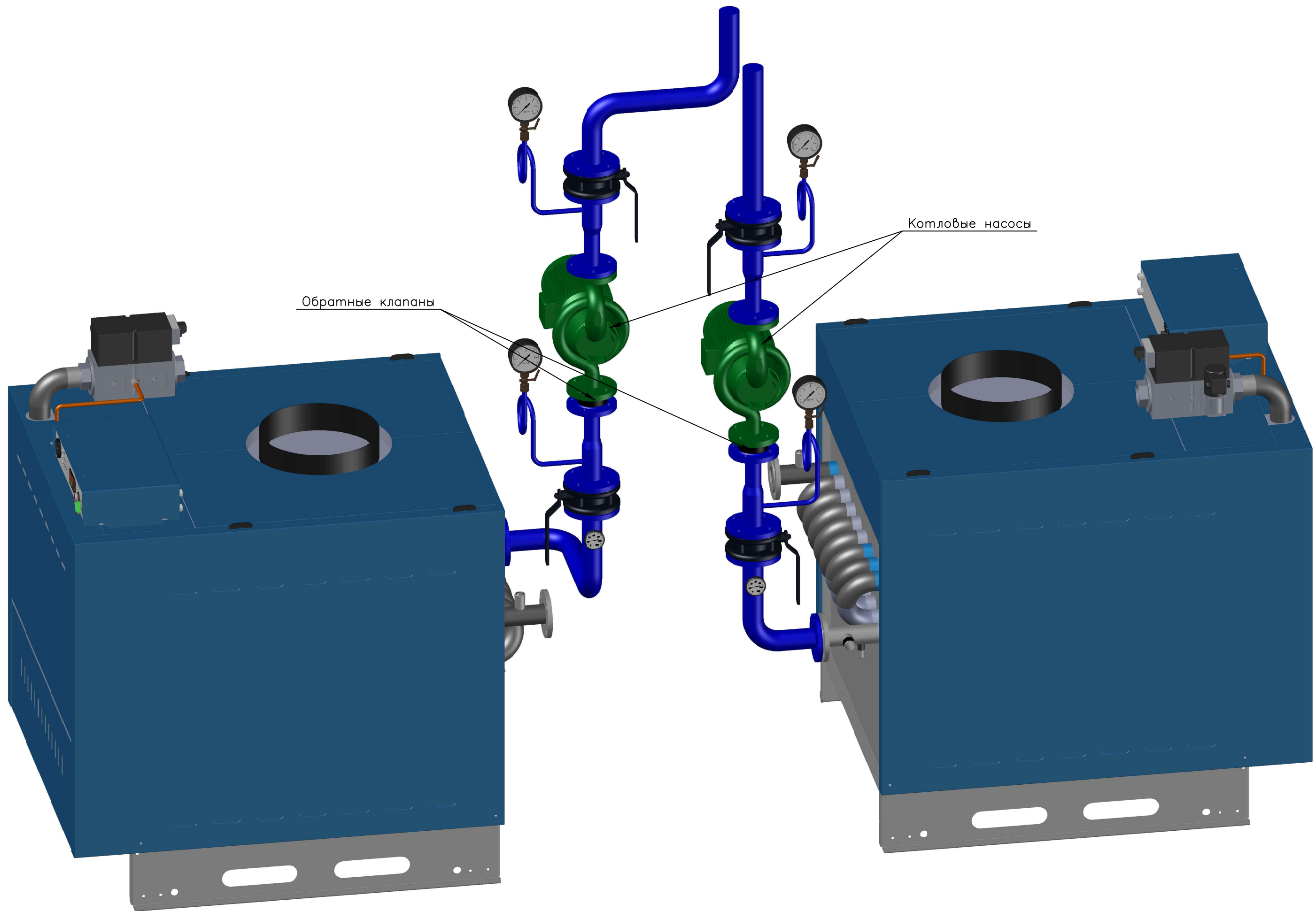
Обратные трубопроводы котлов
