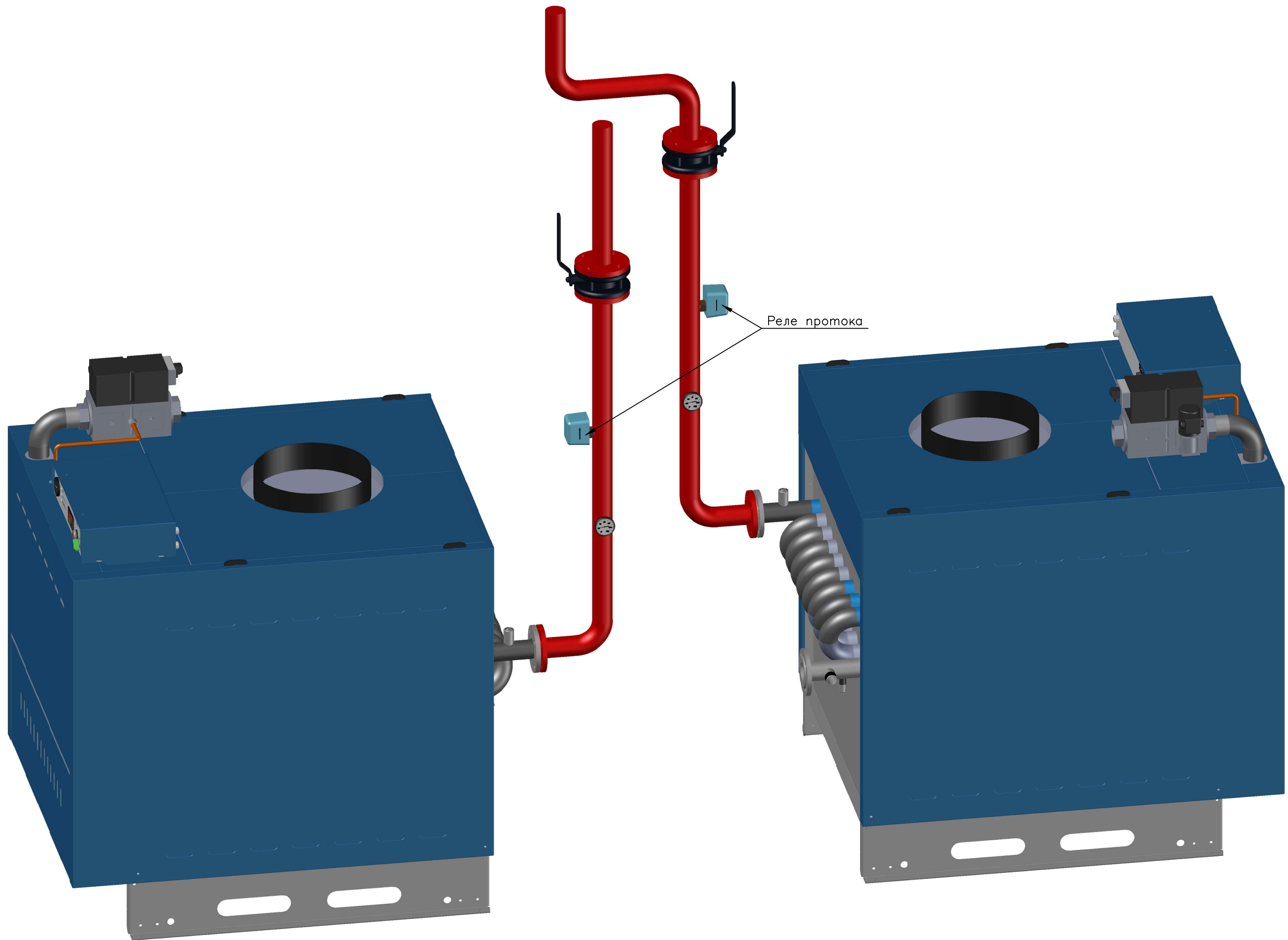
Подающие трубопроводы котлов
